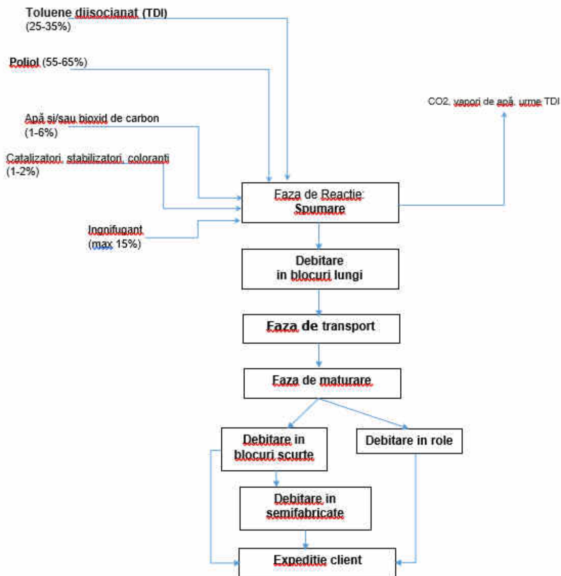
Figura 4 -Descrierea fazelor tehnologice
